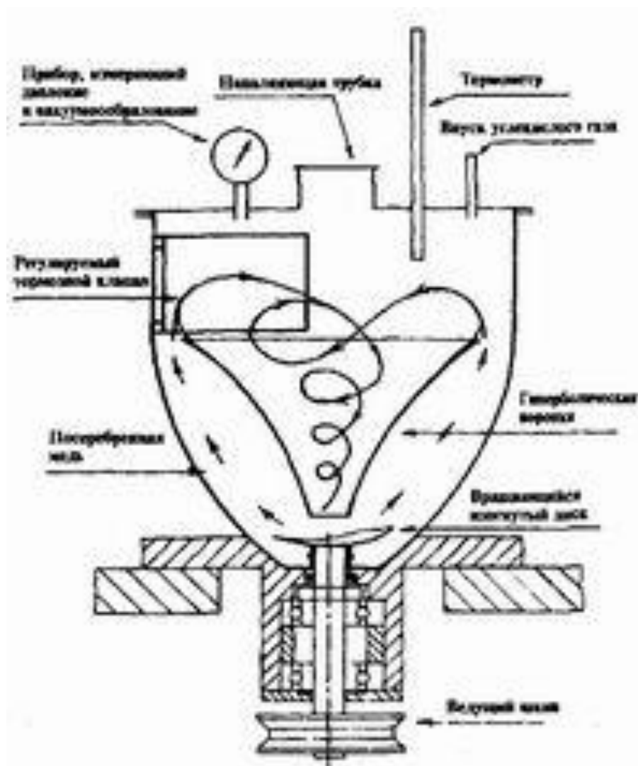
Рис. 25. Репульсатор в разрезе
