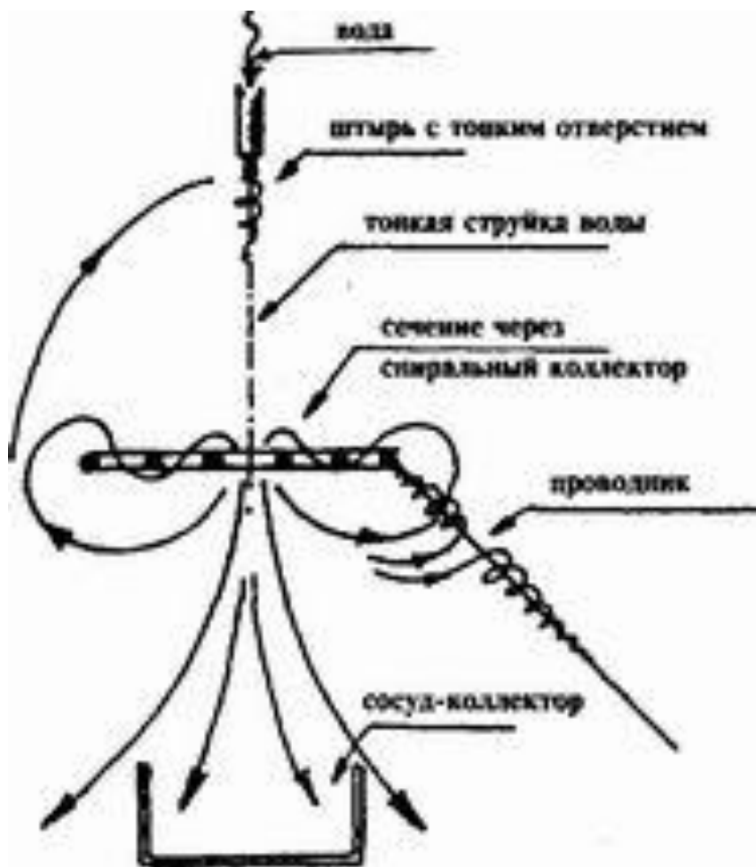
Рис.2 Эксперимент со спирально закручивающейся струей воды. Схематическое изображение прохождения тонкой струи воды по спиралевидному заряженному коллектору
