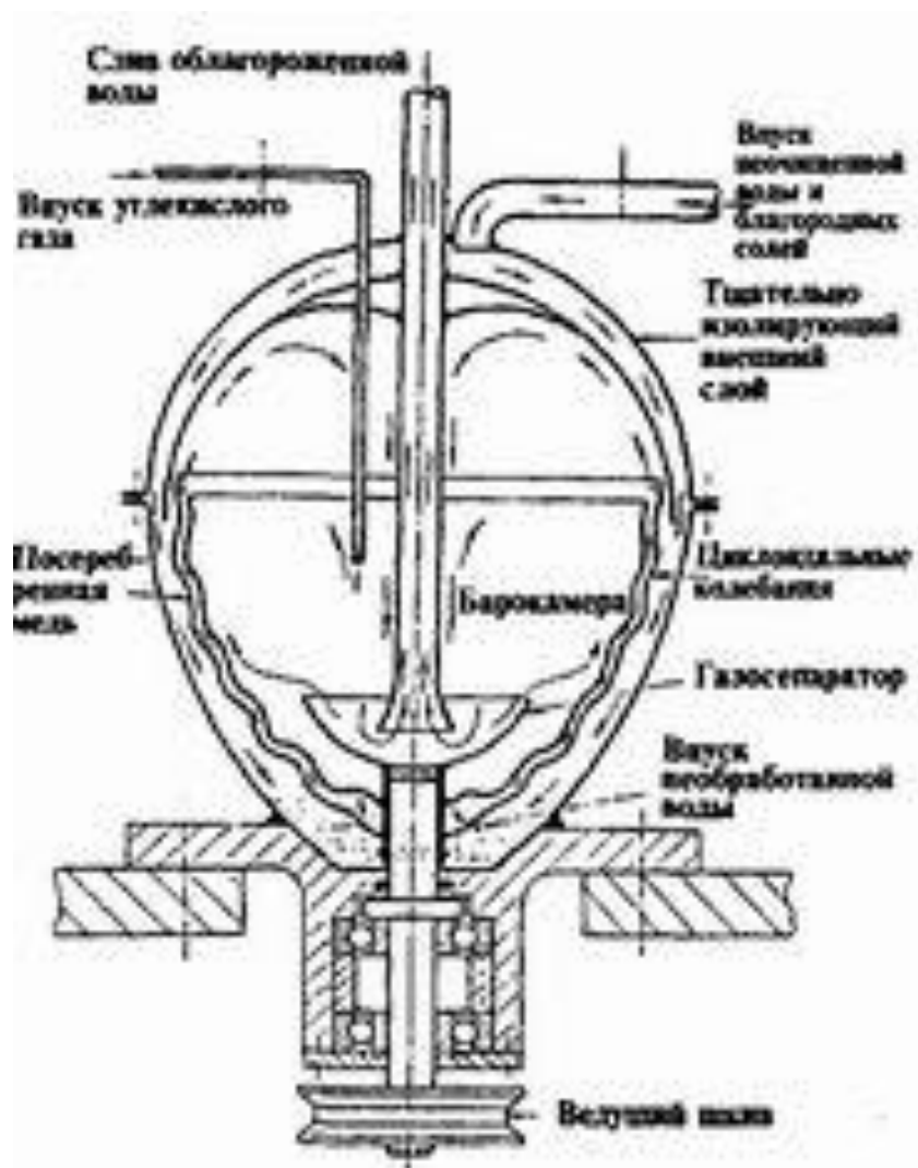
Рис. 24. Принцип устройства репульсатора
