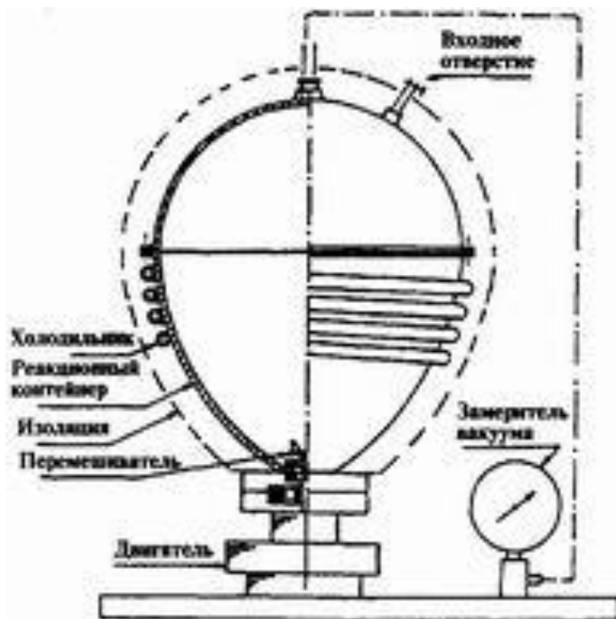
Рис. 26. Схема репульсатора со встроенной охлаждающей установкой Шведский научно-исследовательский институт биологических технологий
