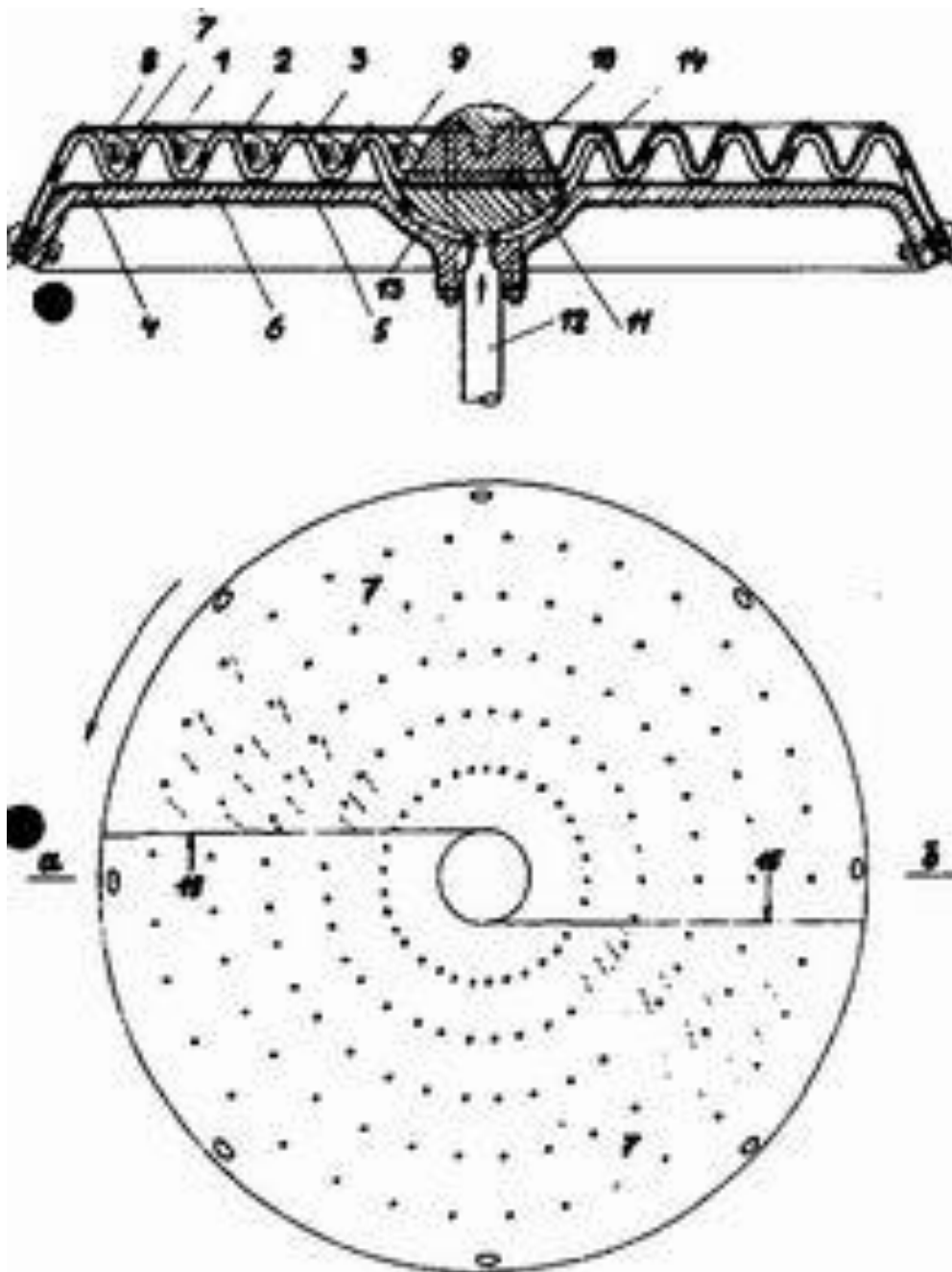
Рис. 30. Репульсив, патент № 146 141
