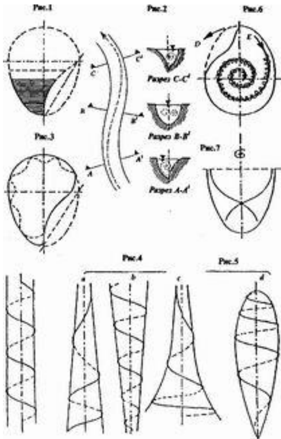
Рис. 18. Чертежи труб с двойной спиральной конфигурацией — иллюстрации к нескольким патентам 6
