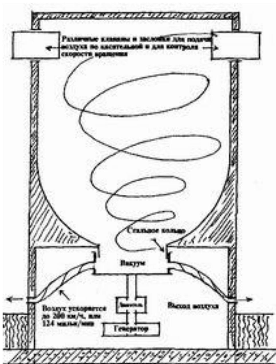
Рис. 21. Импульсионная машина, работающая на воздухе (машина-торнадо — принцип строения)
