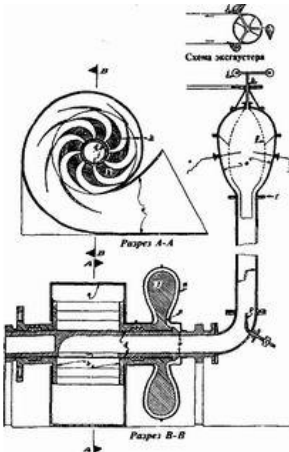
Рис.19. Схема аэротурбины — патент № 145141
